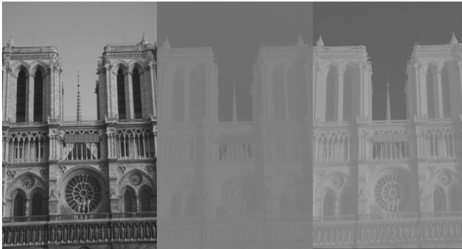
Helligkeit (L-Kanal)
