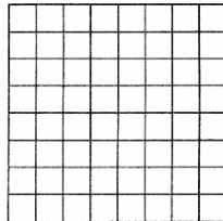
Ortsfrequenz 0
