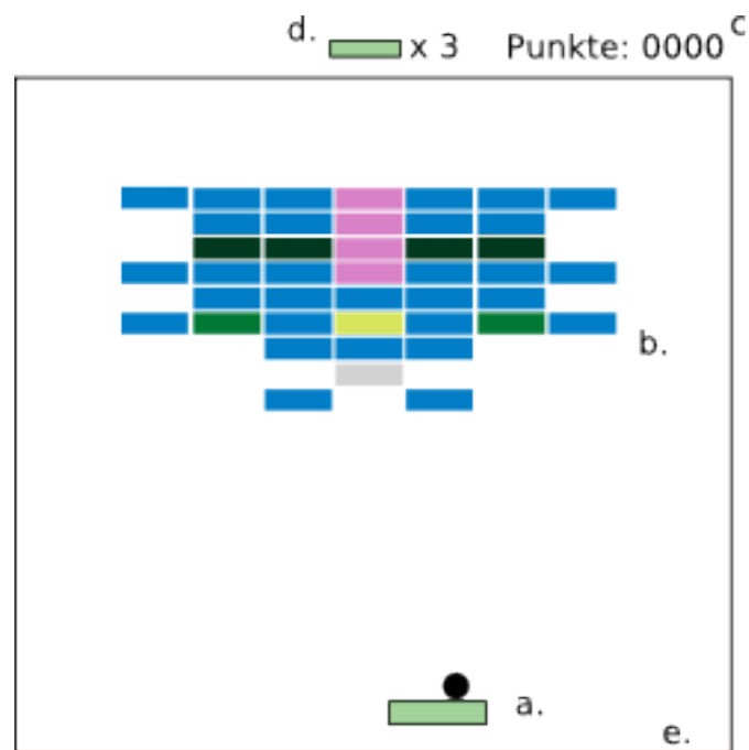
Abbildung 1: Breakout Spielfeld.
